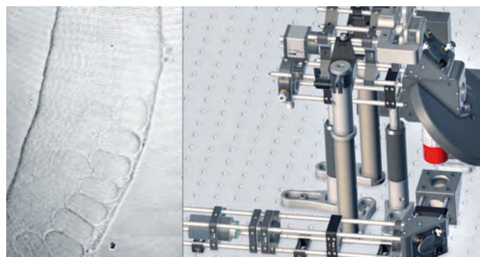
En-face-Aufnahme eines C. elegans Fadenwurms mit seinen Eiern, aufgenommen mit dem VIS-OCT-System (links) und Konstruktion des Fluoreszenzmikroskops kombiniert mit dem Probenarm des OCT-Systems (rechts). Foto: Calvin Kreft & Henrik Thiedig
