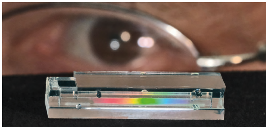
Spektraler Sensor vor dem Auge des Entwicklers. Diese Sensoren müssen klein, kompakt und einfach konstruiert sein und zerlegen das Licht in seine verschiedenen „Farben“; Foto: Aliaksei Kobylinskiy
