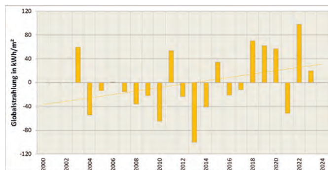
Anomalie Globalstrahlung 2003 bis 2023: Abweichung Jahressummen von mittlerer Jahressumme EAH Jena (1088 kWh/m 2 )
