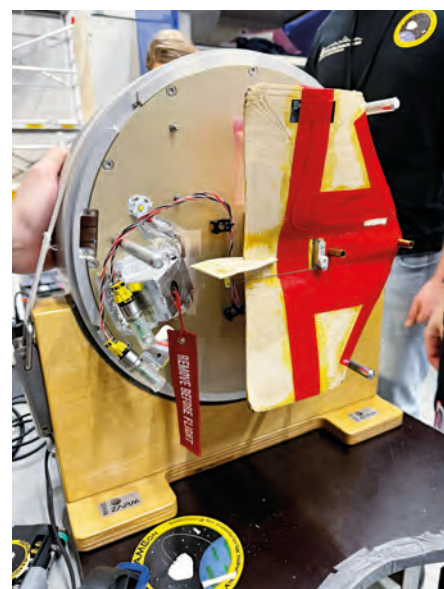
Vollständiges Experiment: Gleiter auf dem Rauswurfmechanismus; Foto: Timon Scheler
