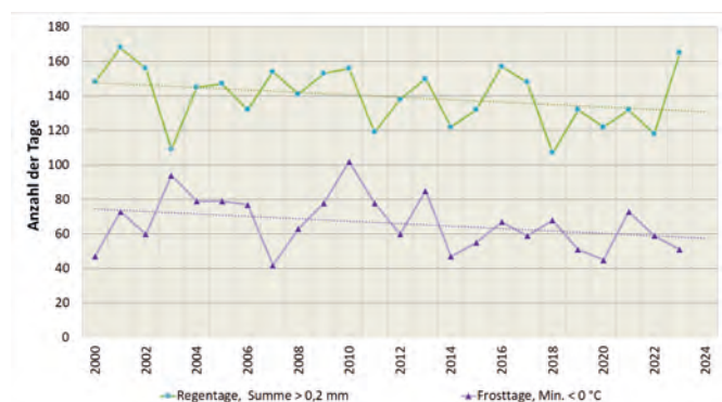
Nach den Daten der EAH Jena von 2000 bis 2023 nehmen Regen- und Frosttage ab.
