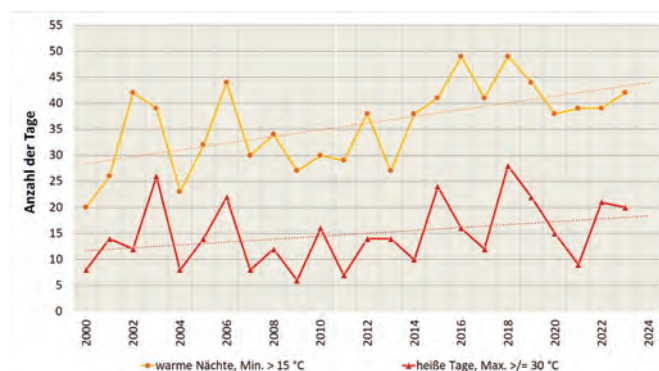
Nach den Daten der EAH Jena von 2000 bis 2023 nehmen warme Nächte und heiße Tage zu. Der Anstieg bei den warmen Nächten ist höher.
