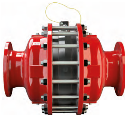
Flammdurchschlagsicherung (Detonationsrohrsicherung), bis max. Anschlussnennweite DN1000 (Flammenfilterdurchmesser 2000 mm), für Wasserstoff (IIC) bis max. DN250; Copyright: Braunschweiger Flammenfilter GmbH (PROTEGO)
